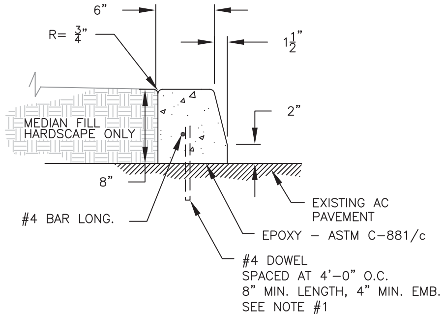
A MEDIAN CURB - TYPE A3 N.T.S
